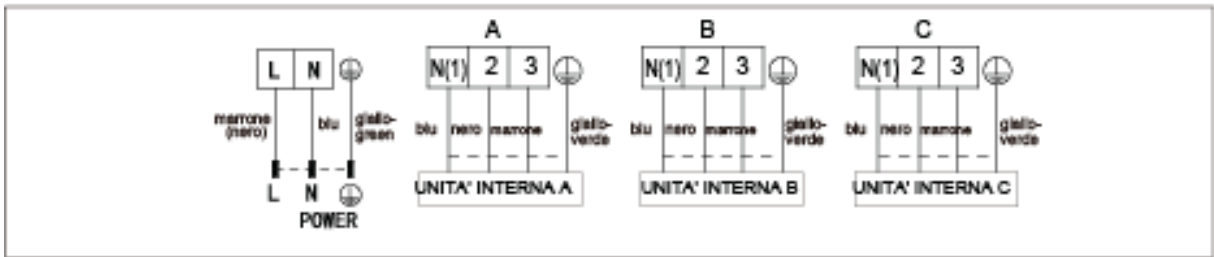
All'alimentazione elettrica
