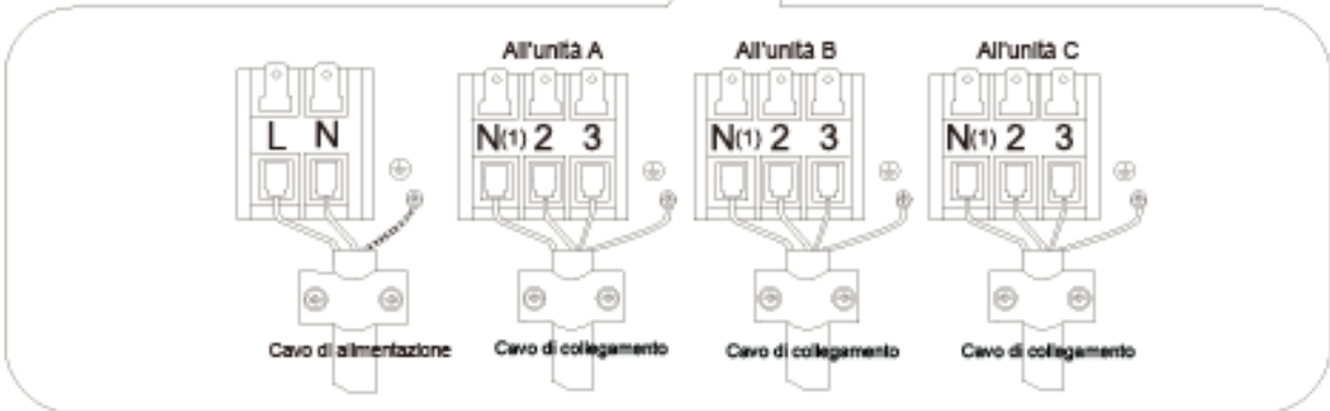
All'alimentazione elettrica
